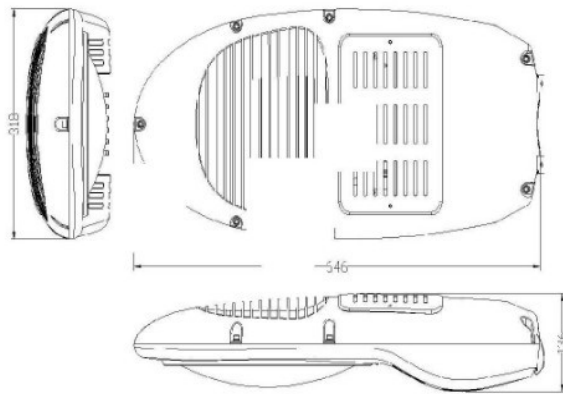
尺寸图
